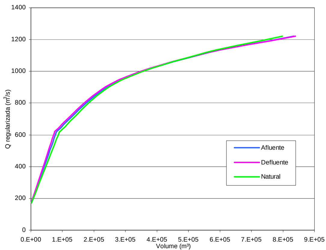
Figura 3 - Curvas de regularização no período de 1980 a 2003 – Usina Salto Santiago
